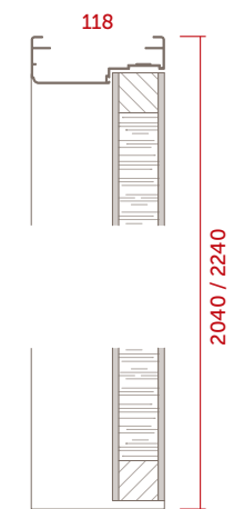
MARCO DE ALUMINIO
