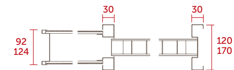
MARCO DE CHAPA
