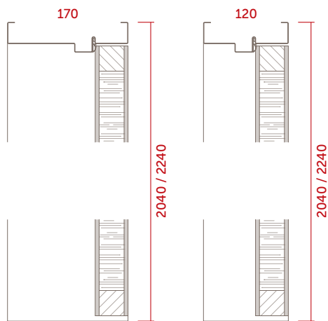
MARCO DE CHAPA
